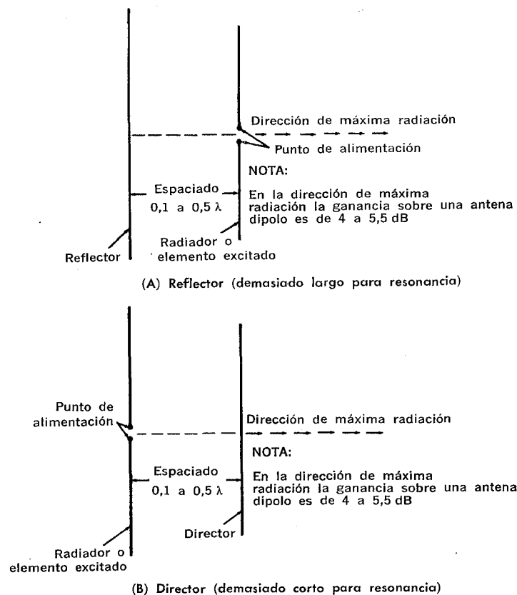
Fig. 3-9. Antenas direccionales de dos elementos.
