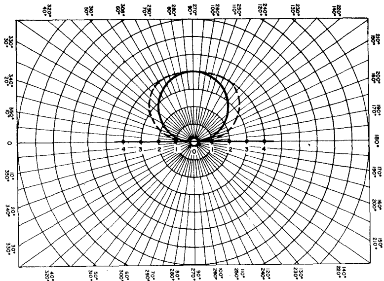
(A) 0,1 (línea llena) y 0,25 (línea de trazos), longitudes de onda sobre el terreno
