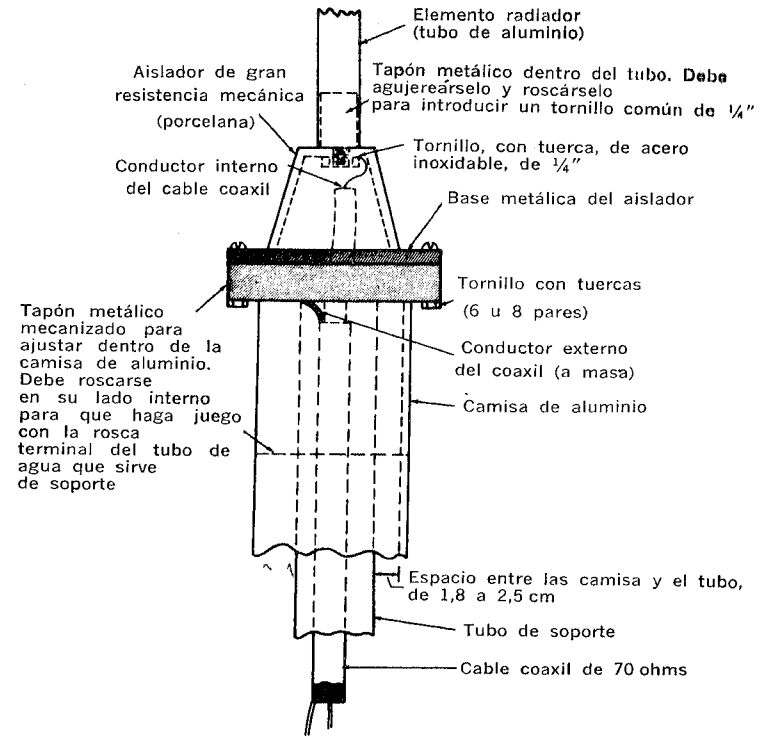
Fig. 3-31. Detalles de la estructura del punto de alimentación.
