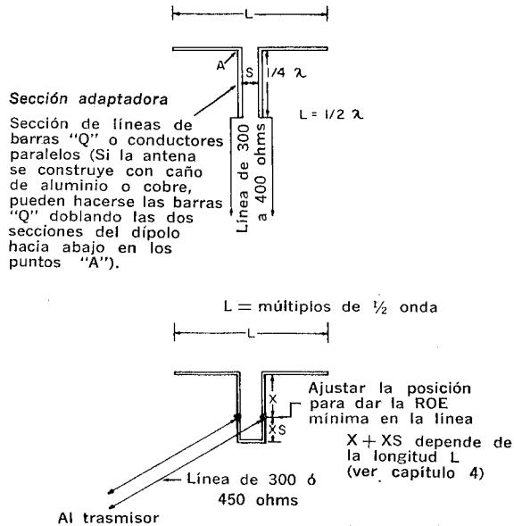
Fig 7-31. Adaptación de una línea de conductores paralelos de 300-400 ohms al elemento excitado.
