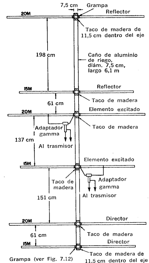
Fig. 7-26. Antena de elementos entrelazados para 15 y 20 metros (para las longitudes consultar la Tabla 7-1).
