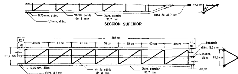
Fig. 8-1. Torre de comunicaciones de uso general.
