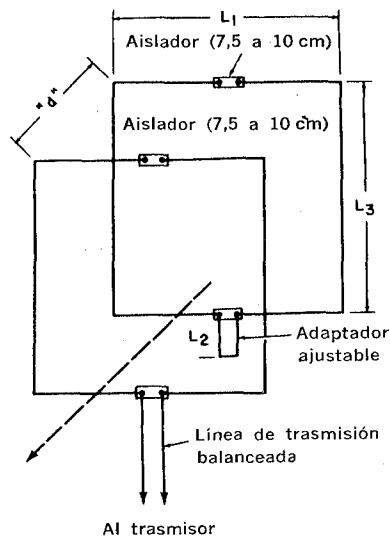
Fig. 3-24. Antena cuádrlica cúbica de media onda.
