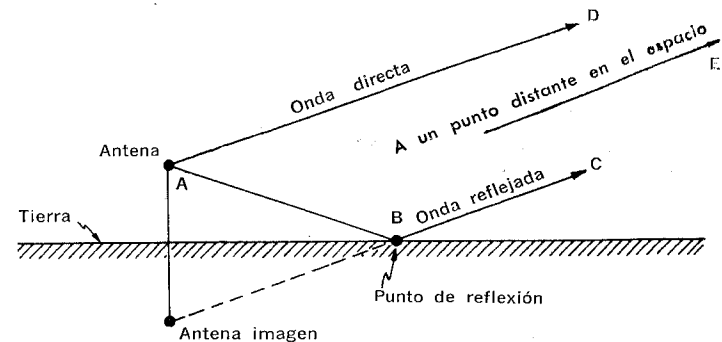
Fig. 2-9. Ondas directa y reflejada provenientes de una misma antena.
