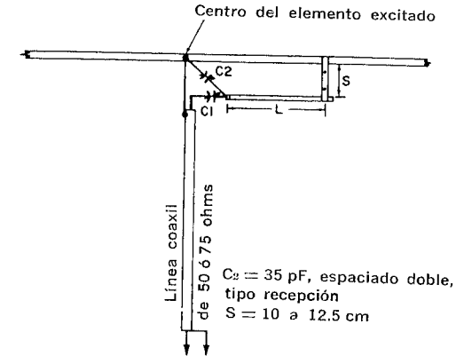
Fig. 5-16. El adaptador gamma modificado.
