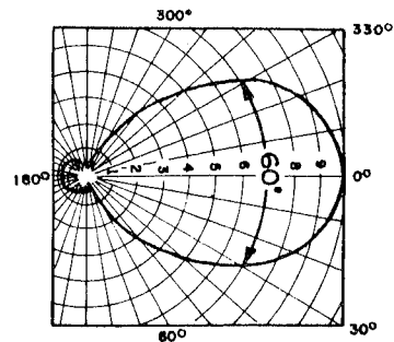
DIAGRAMA POLAR TÍPICO EN 10, 15 Y 20 METROS
