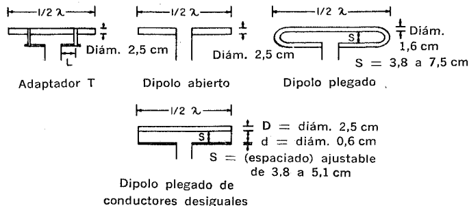
Fig. 7-30. Elementos excitados para antenas de FME (VHF).
