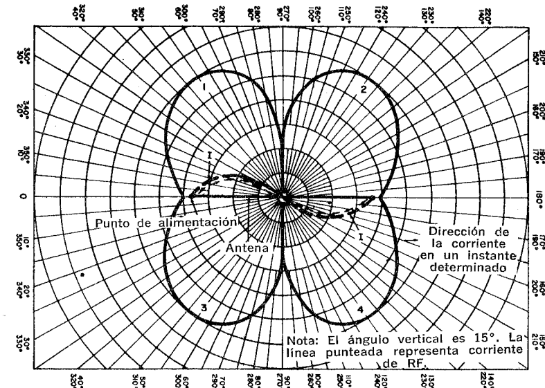
Fig. 3-2. Diagrama de irradiación de una antena de onda completa alimentada en un extremo.
