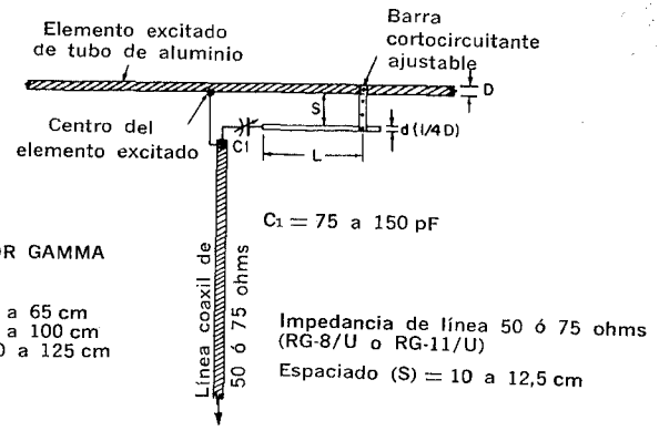
Fig. 5-13. Adaptador gamma.
