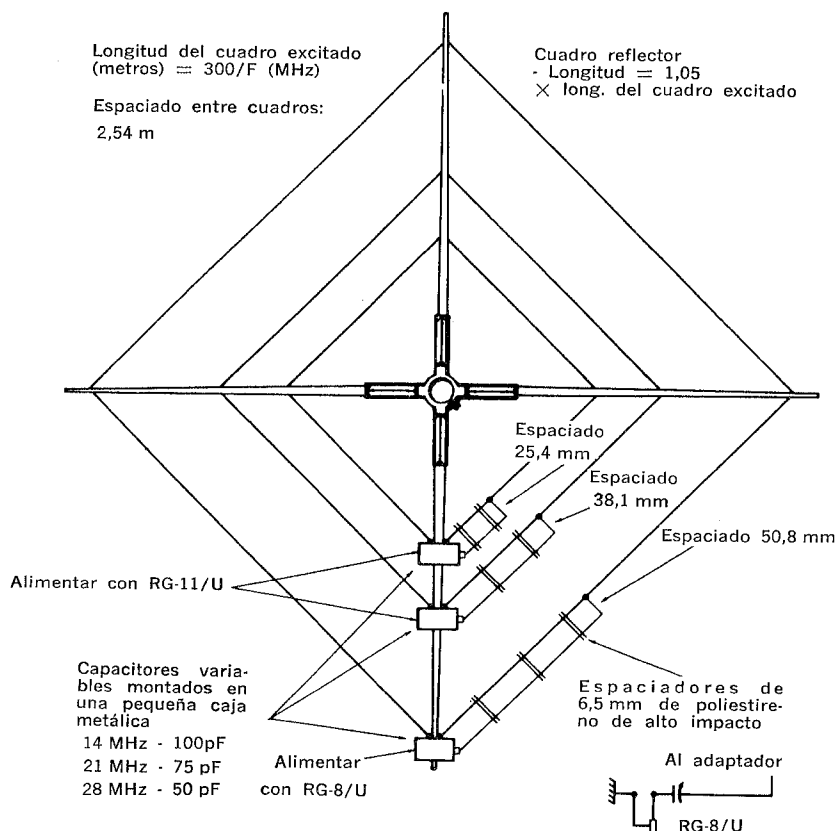
Fig. 7-21. Antena cuádrada de dos elementos, alimentada en "rombo" y con adaptadores gamma para 14, 21 y 28 MHz.
