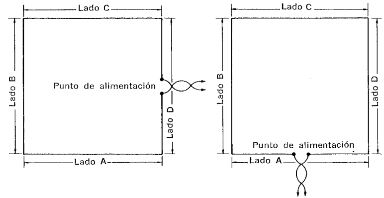
(A) Emisión polarizada verticalmente (alimentada en el centro del lado "D")
