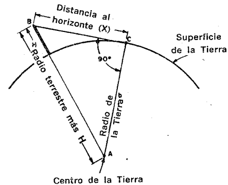
Fig. 1-4. Cálculo geométrico de la distancia al horizonte de una antena.
