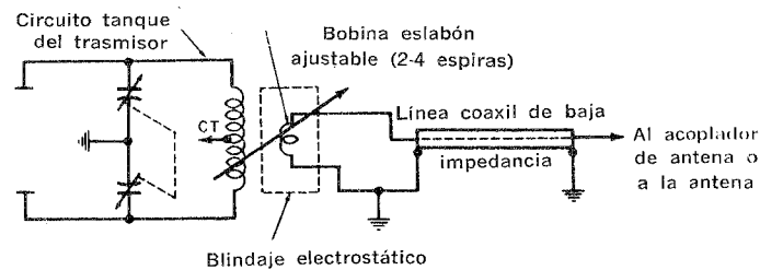
(A) Simétrico (push-pull)
