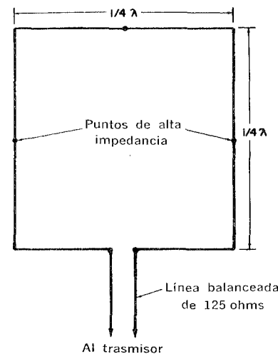
Fig. 3-22. Cuadro básico de las antenas cuádricas.
