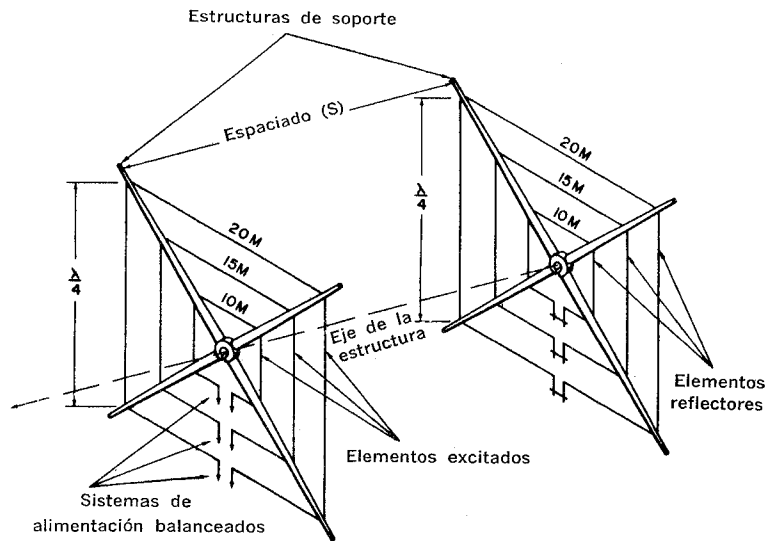
Fig. 7-9. Antena cuádrlica multibanda con una sola estructura de soporte.
