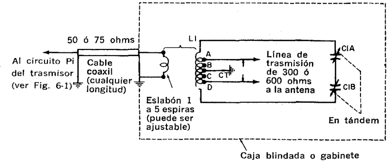
Fig. 6-2. Acoplador de antenna para adaptar una salida desbalanceada de baja impedancia a líneas simétricas de 300-600 ohms.
