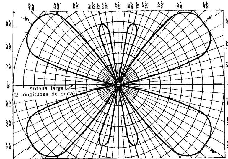
Fig. 3-4. Diagrama de irradiación de una antena de dos ondas completas.
