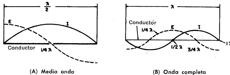
Fig. 3-1. Tensión y corriente de radiofrecuencia en antenas lineales.
