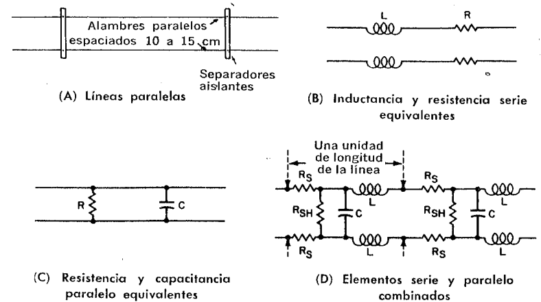
Fig. 4-4. Constantes RLC distribuidas en una línea de transmisión.
