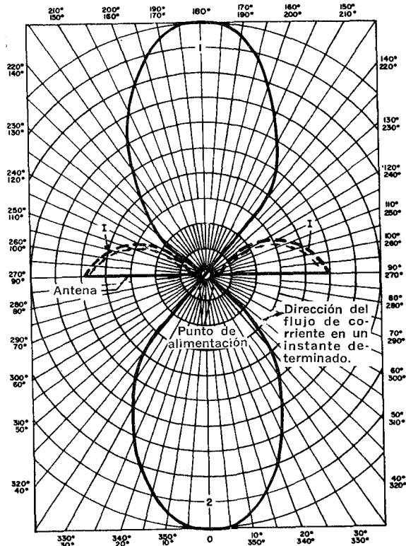
Fig. 3-3. Diagrama de irradiación de una antena de onda completa alimentada al centro.
