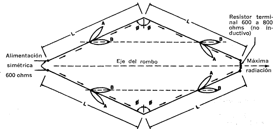
Fig. 3-7. Antena rómbica.
