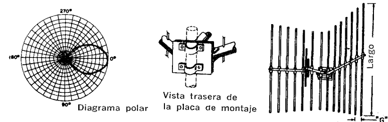
Fig. 3-34. Antena comercial con reflector esquinero.
