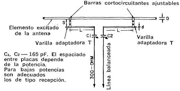
Fig. 5-12. Uso de capacitores para cancelar la inductancia de la sección T.
