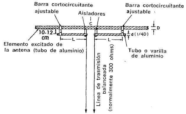
Fig. 5-11. Adaptador T.
