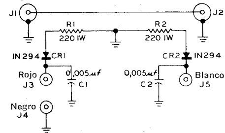
Fig. 6-8. Circuito del acoplador direccional de la Johnson.
