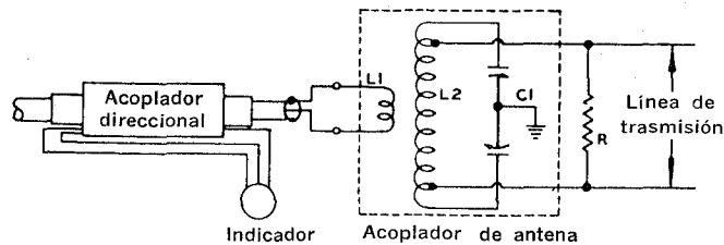
Fig. 6-11. Acoplador direccional e indicador utilizados con un acoplador de antena.
