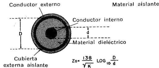
(D) Cable coaxil
