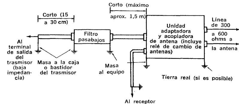
Fig. 6-3. Conexión del filtro pasabajos con el acoplador de antenna.
