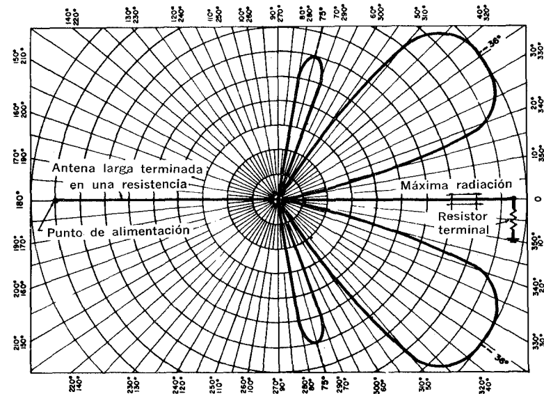
Fig. 3-5. Diagrama de irradiación de una antena larga alimentada en un extremo y terminada en Z_0 .
