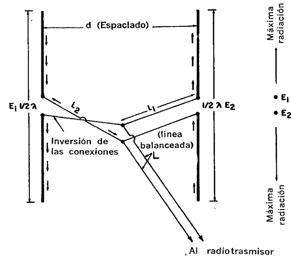
Fig. 3-13. Antena activa con dos elementos de media onda alimentados fuera de fase.
