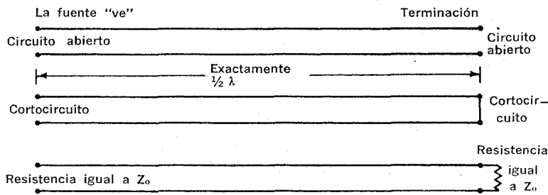
Fig. 4-10. Características de líneas de transmisión que son múltiplos exactos de media onda.
