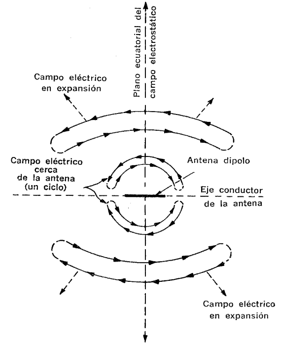
Fig. 2-3. Campo eléctrico alrededor del conductor de una antena.
