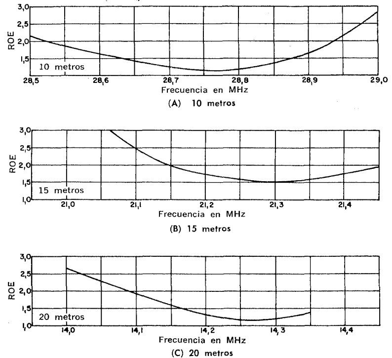
Fig. 7-5. Curvas de ROE para la antena Mosley TA-36.
