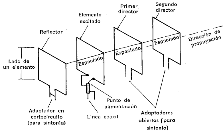
Fig. 7-8. Configuración cuádrlica típica de 4 elementos.
