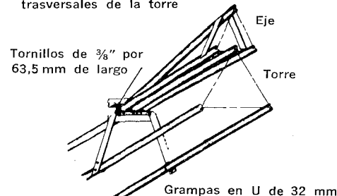
(B) Grampa de anclaje
