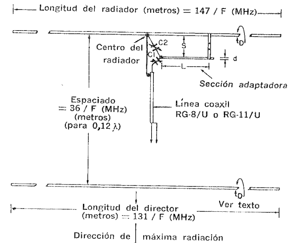
Fig.7-1 Antena parasitaria sencilla de dos elementos.
