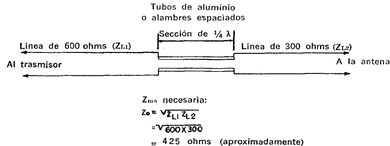
Fig. 5-3. Sección de cuarto de onda utilizada para adaptar líneas desiguales.
