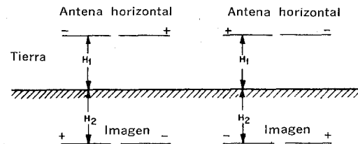
Fig. 2-11. Dipolos de media onda y sus imágenes.
