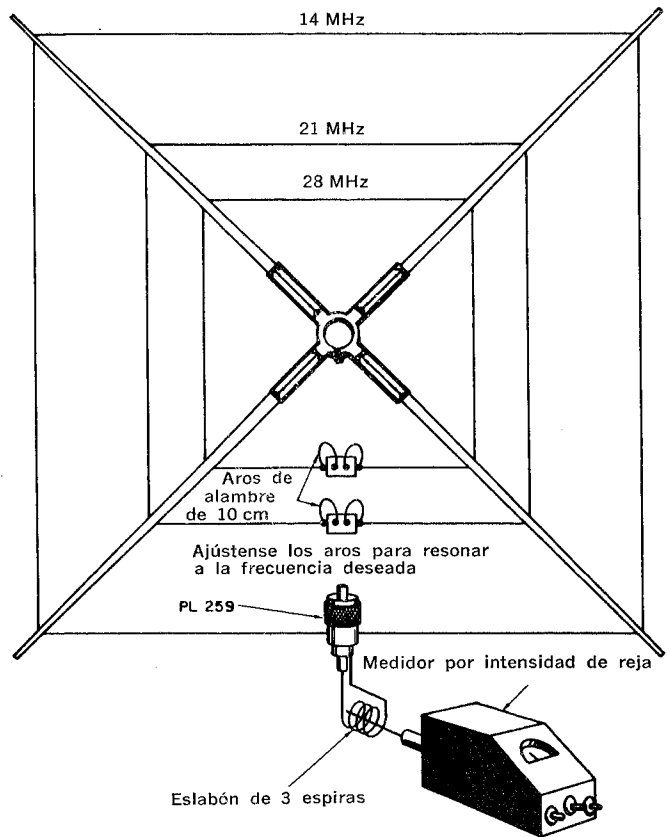
Fig. 7-23. Medición de la resonancia del elemento excitado en la antena.
