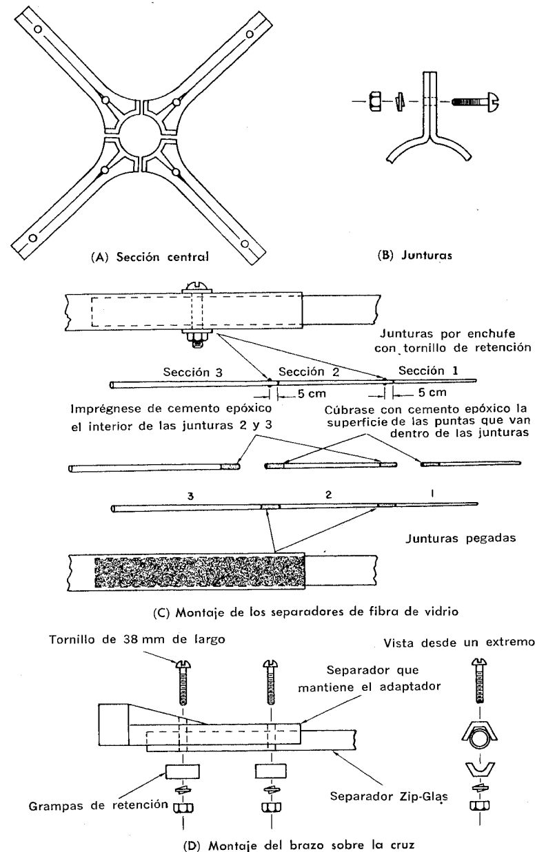
Fig. 7-11. Dispositivo de montaje Starmount de Polygon.
