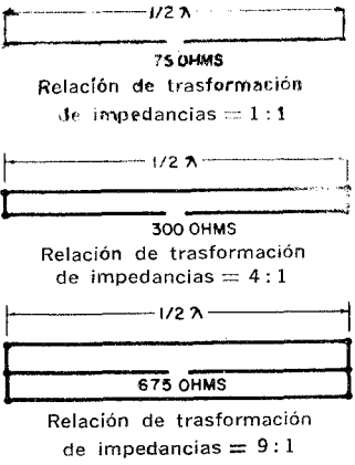
Fig. 5-10. Aumento de la impedancia del punto de alimentación de una antenna de media onda mediante el agregado de conductores.
