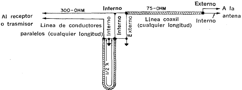
Fig. 5-9. Balún de media onda para adaptar una antenna de 75 ohms a una línea de trasmisión de 300.
