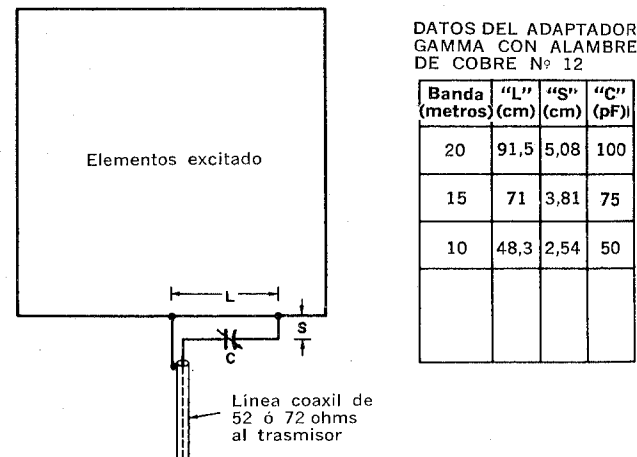
Fig. 7-22. Dimensiones y valores de los capacitores para las secciones gamma de la Fig. 7-21.
