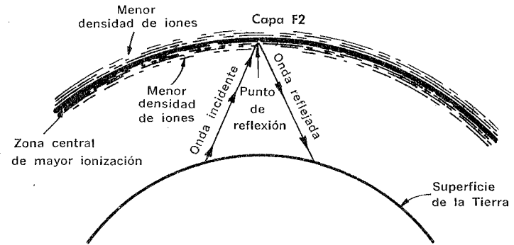
Fig. 1-8. Refracción ionosférica.
