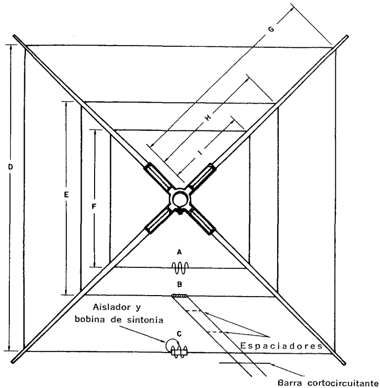
DATOS DEL REFLECTOR Y DIRECTOR (Medidas en pulgadas)
