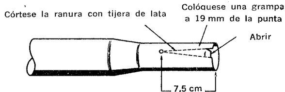
(B) Extremo ahusado
