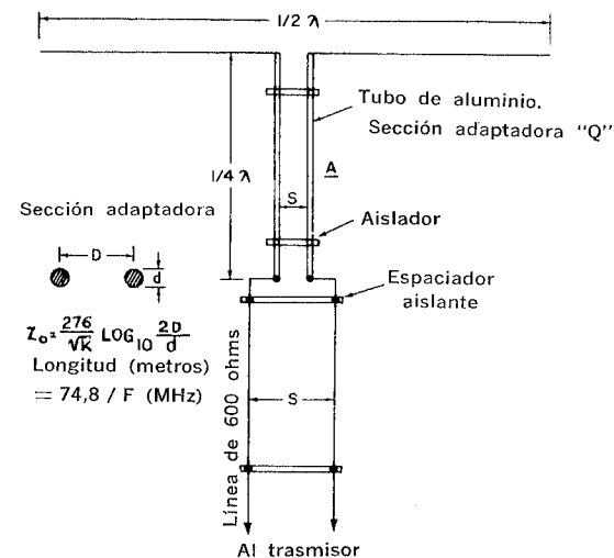
Fig. 5-2. Sección adaptadora hecha con tubos de aluminio para transmisores de alta potencia.
